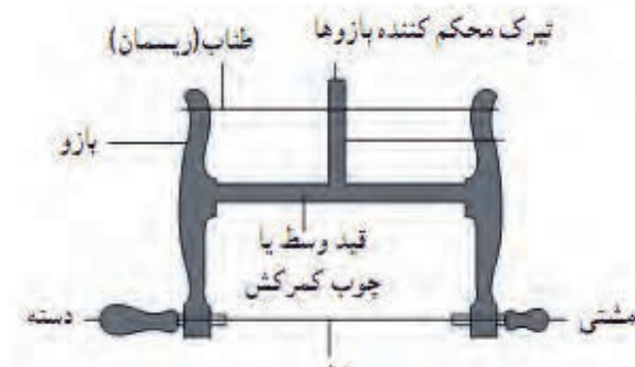
شکل ۵-۵- قسمت‌های مختلف ارّه کلافی.
