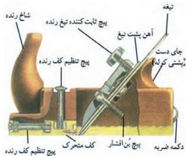
شکل ۶-۲- قسمت‌های مختلف رنده‌ی دستی چوبی.
