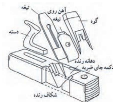
شکل ۶-۱۳- قسمت‌های مختلف اجزای رنده پوبی و نحوه‌ی جاگذاری آنها.
