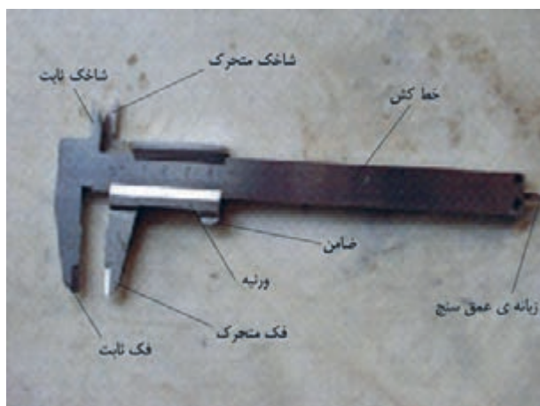
شکل ۱۴-۳۰ - کولیس ساده.
