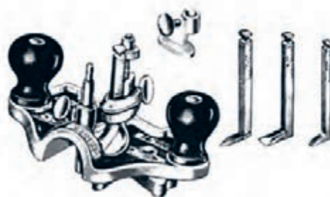
شکل ۶-۴۱ رنده‌ی کفِ طرح فرنگ همراه تیغه‌ها.
