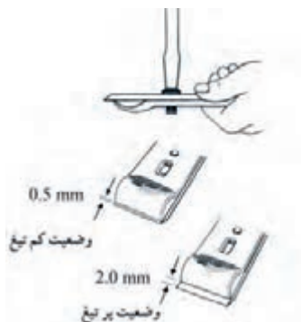
شکل ۶-۶۵- تنظیم و محکم کردن تیغه و پشت‌بند.
