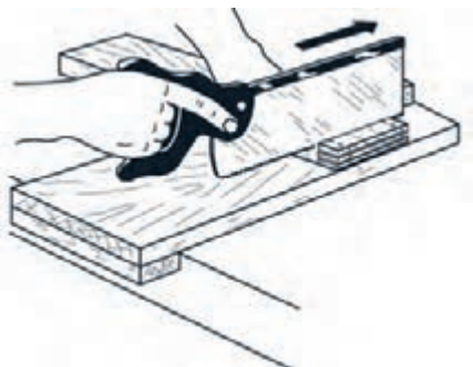
شکل ۵-۵۶. بریدن قسمت‌های اضافی (بر انداختن زبانه).
