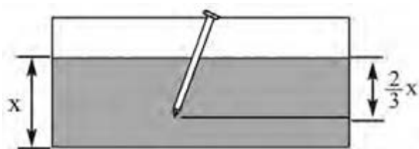
شکل ۷-۲۹- نسبت طول میخ با قطعه کار.
