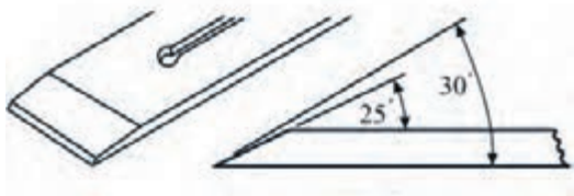
شکل ۶-۸- زاویه‌ی پخ تیغه رنده.
