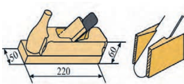
شکل ۶-۲۵. ابعاد کوله‌ی رنده قاجی و نمونه‌ی قرار گرفتن تیغه داخل کوله.
