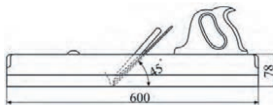
شکل ۵۰-۶- ابعاد رنده بلند و زاویه‌ی قرار تیغه‌ی آن.
