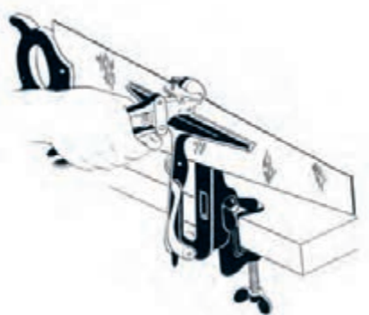
شکل ۱۴-۵۶- انجام عمل چپ و راست کردن به وسیله انبر چپ و راست کن.
