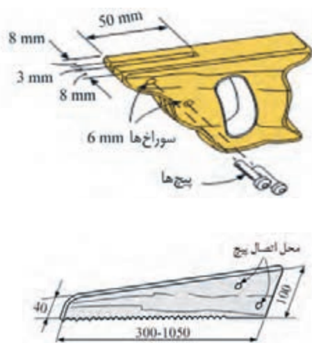
شکل ۵-۷- تیغه ارّه دُم روباهی.
