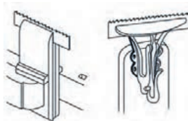
شکل ۱۴-۲۷- بستن تیغه اره در داخل تنگ اره تیزکنی.
