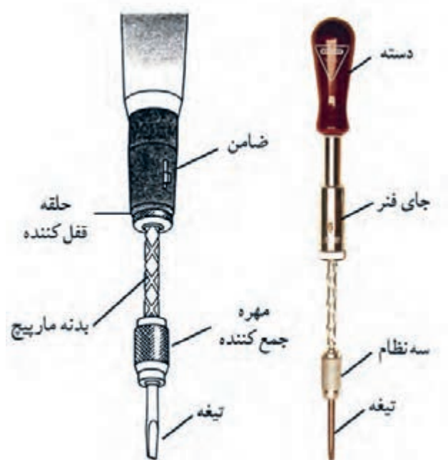
شکل ۱۲-۷. قسمت‌های مختلف یک دریل فشاری.
