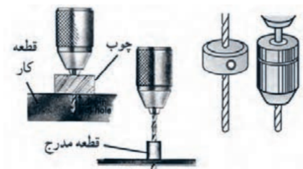
شکل ۱۲-۳۹. چند نوع عمق سنج دریل.
