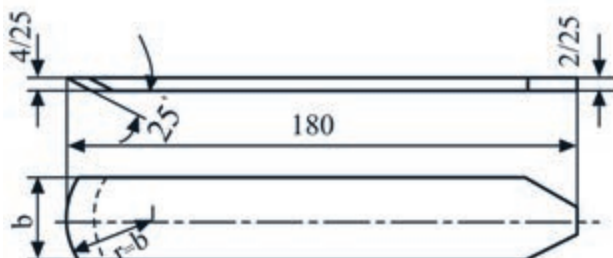
شکل ۶-۲۴. تیغه‌ی رنده قاجی.
