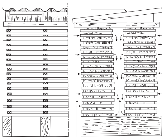
شکل ۳-۴۲- نمونه‌ی دستک‌گذاری و استفاده از سقف ایرانی.
