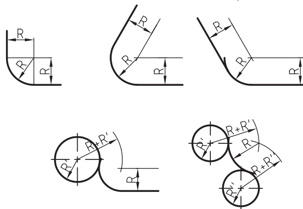
شکل ۱۵-۴۲- برخی از قوس‌های لبه‌ی کار یا پروفیل‌ها.
