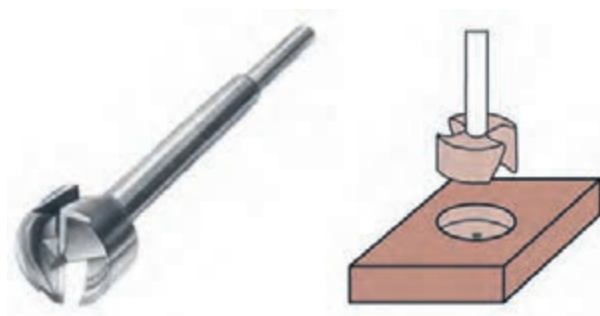
شکل ۱۲-۲۶- سر مته‌ی مرکزی و کاربرد آن.
