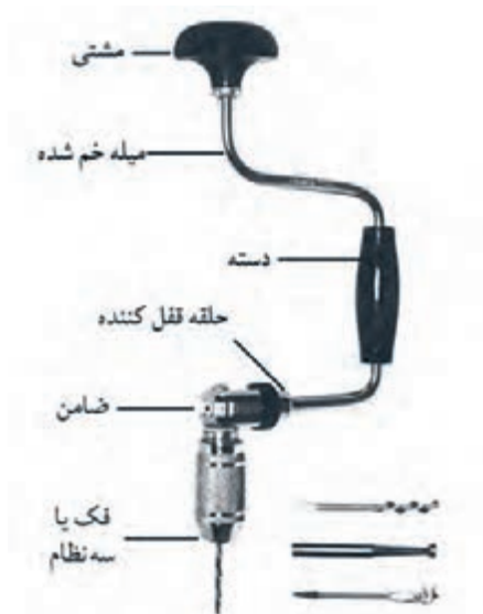
شکل ۱۲-۱- قسمت‌های مختلف دریل شتر گلو، همراه با چند سر مته با دنباله‌های مختلف.
