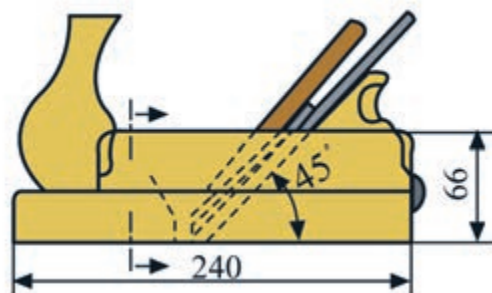
شکل ۶-۲۶- زاویه‌ی قرار تیغه‌ی رنده قاجی.
