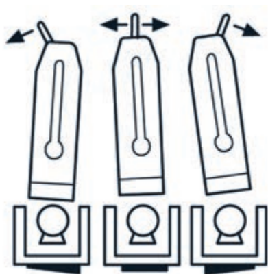
شکل ۶-۶۶- تنظیم تیغه رنده به کمک اهرم جانبی.
