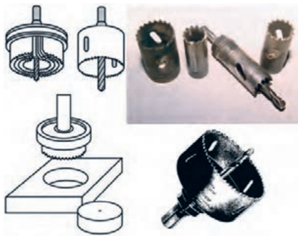
شکل ۱۲-۲۸. سر مته‌ی گردبر و کاربرد آن.
