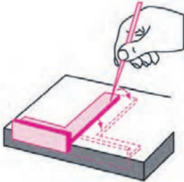
شکل ۹۹-۴. آزمایش گونیا‌یی بودن گونیا.
