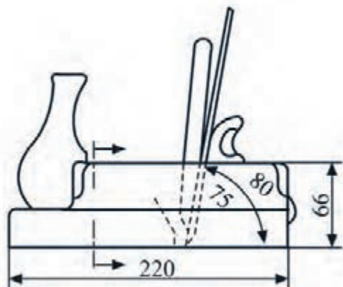
شکل ۵۲-۶- ابعاد رنده فشی و زاویه‌ی قرار تیغه‌ی آن.
