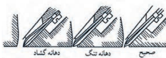
شکل ۶-۱۴- دهانه‌ی کف رنده در سه وضعیت.
